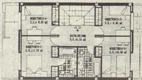
PLANTA PRIMERA
