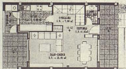
PLANTA BAJA
