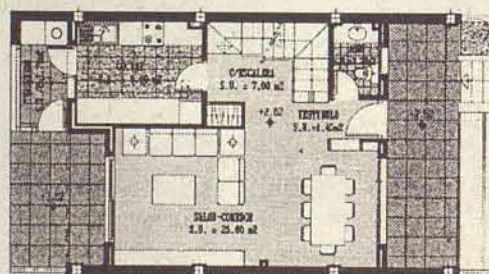
PLANTA BAJA
