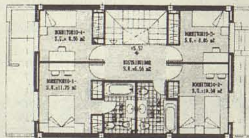
PLANTA PRIMERA
