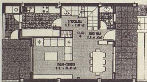
PLANTA BAJA
